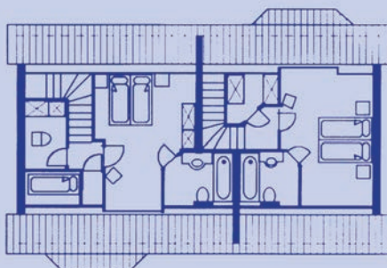
Grundriss Dachgeschoss
